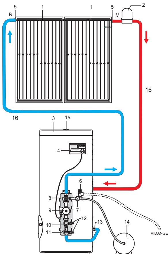
Régulation différentielle incluse SOL
